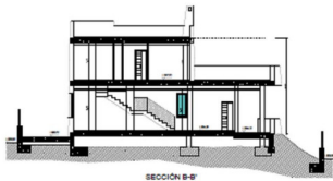
SECCIÓN B-B'
