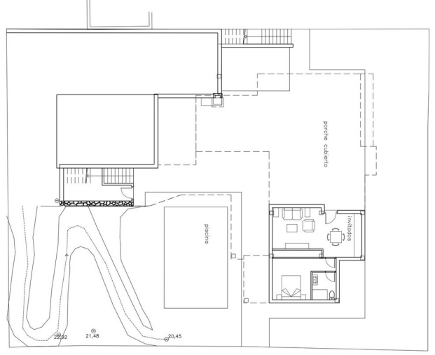
ANTERPROYECTO DE VIVIENDA UNIFAMILIAR NIVEL 2
