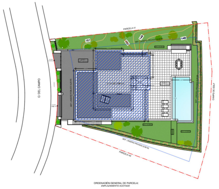
ORDENACIÓN GENERAL DE PARCELA: EMPLAZAMIENTO ACOTADO
