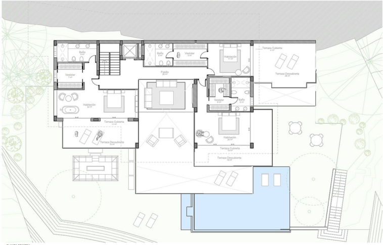
PLANTA PRIMERA 1:100
