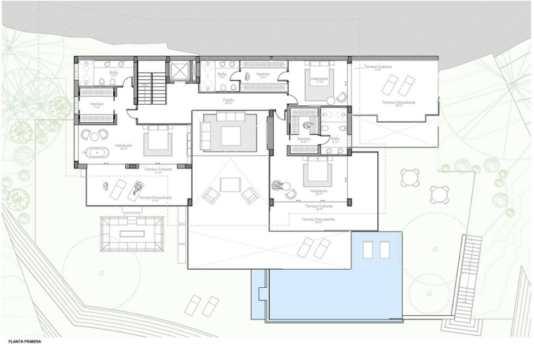
PLANTA PRIMERA 1:100
