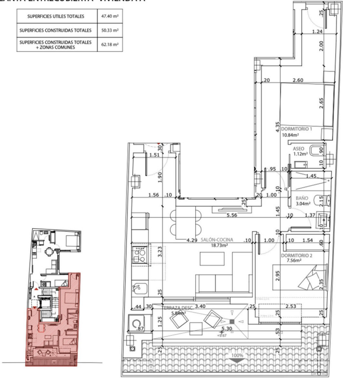
PLANTA ENTRECUBIERTA -VIVIENDA A
