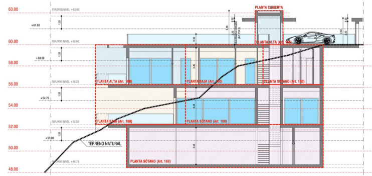
SECCION
