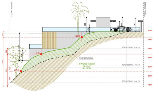
ALZADO NORTE
