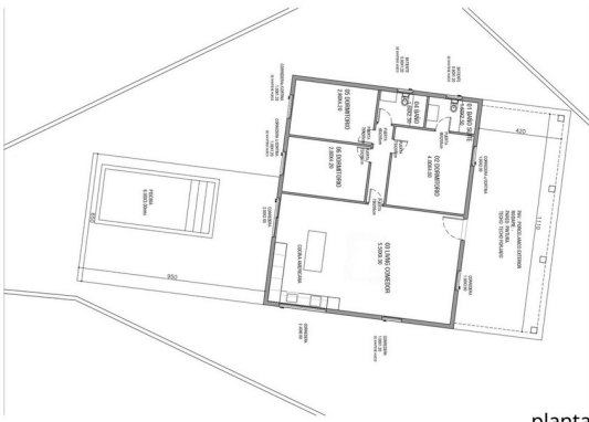
planta propuesta
