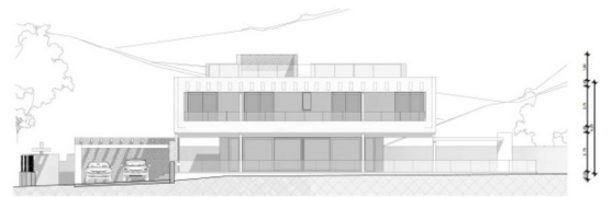
ALZADO SUROESTE
