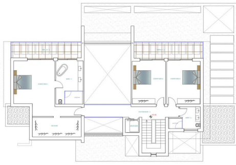
PLANTA ALTA
