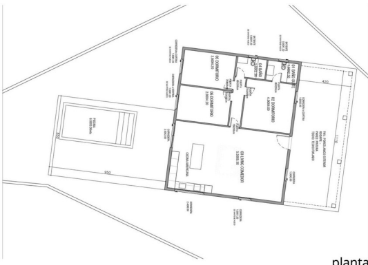
planta proposta
