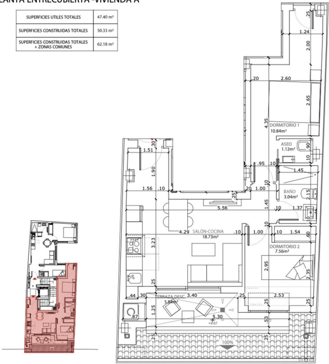
PLANTA ENTRECUBIERTA -VIVIENDA A
